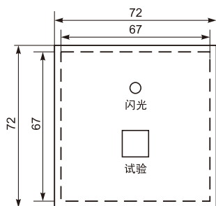
前视图
