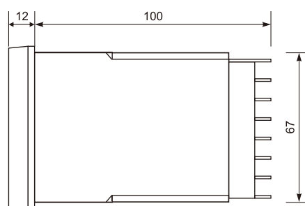
侧视图
